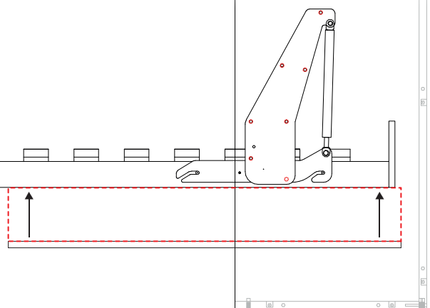
Схема закріплення фасадів
