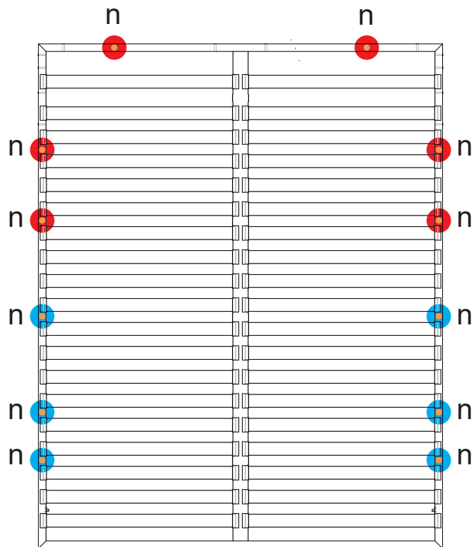
Схема закріплення фасадів
